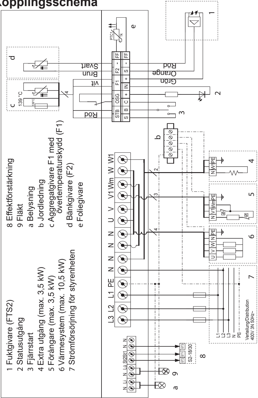
Bild10 Kopplingschema
