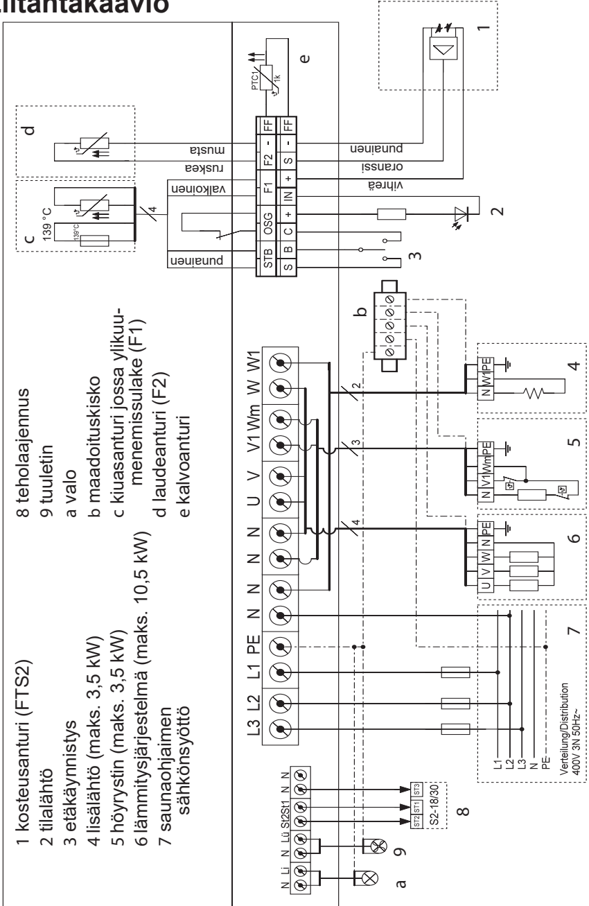
Kuva 10 Liitäntäkaavio
