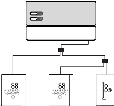
Kuva9 Liitäntäesimerkki Pro D3i
