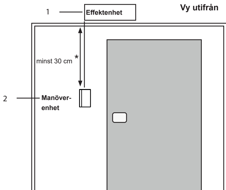
Bild4 Position manöverenhet
