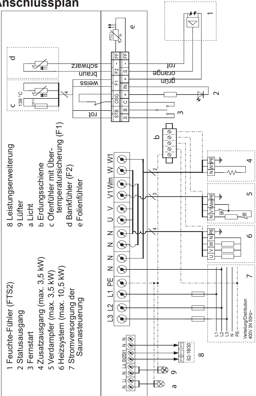
Abb. 10 Anschlussplan
