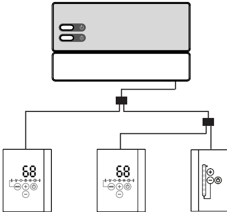
Bild9 Anslutningsexempel Pro D3i
