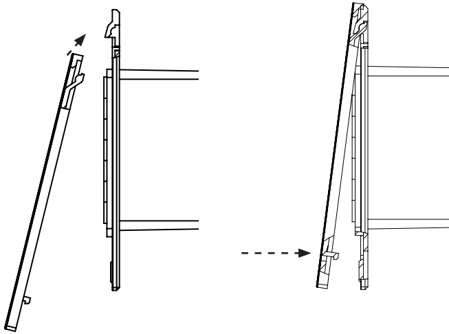
Kuva7 Hallintalaitteen asennus
