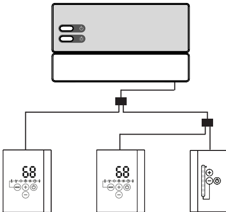
Afb.9 Aansluitvoorbeeld Pro D3i
