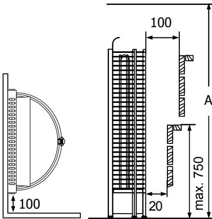
Kuva 2 | Minimisuojaetäisyydet (mm) Fig. 2 | Minimum safety distances (mm)
