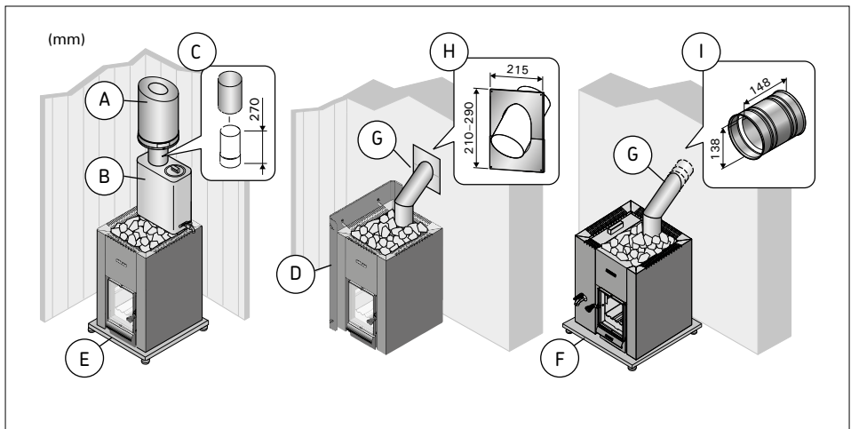
Kuva 16. Lisätarvikkeet. Mitat millimetreinä. Bild 16. Tilläggsutrustning. Måtten i millimeter.
