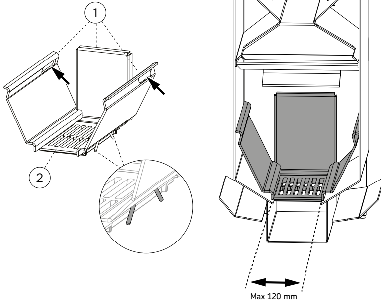
Kuva 2. Palamisilmanohjaimet.
