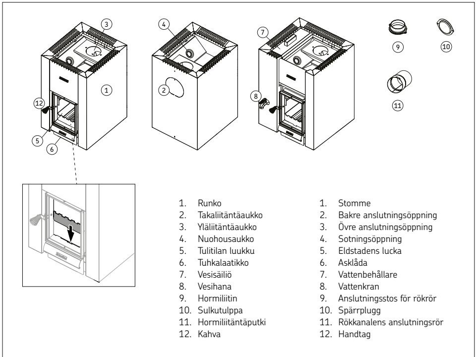
Kuva 1. Kiukaan osat.
