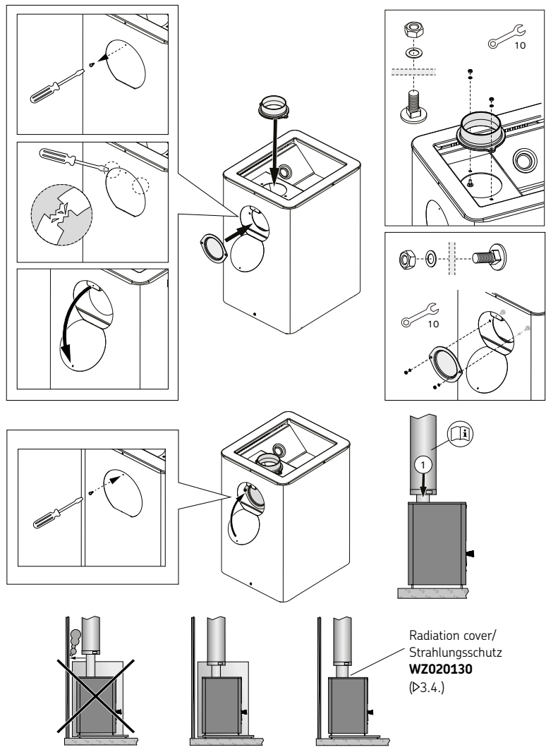
Figure 13. Connecting the stove to a Harvia steel chimney. Abbildung 13. Anschluss des Ofens an einen Harvia-Edelstahlschornstein.
