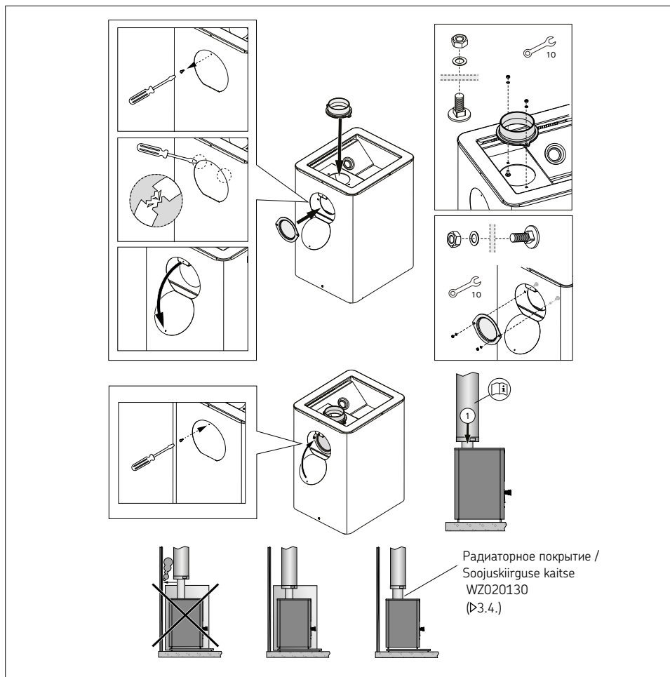
Рисунок 13. Присоединение печи к стальному дымоходу Harvia. Joonis 13. Kerise ühendamise Harvia teraskorstnaga
