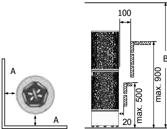
Kuva 2 | Minimisuojaetäisyydet (mm) Fig. 2 | Minimum safety distances (mm)
