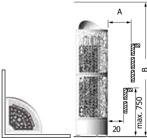
Kuva 2 | Minimisuojaetäisyydet (mm) Fig. 2 | Minimum safety distances (mm)
