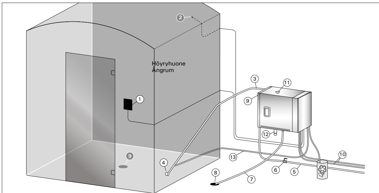
Kuva 1. Höyrykehittinjärjestelmän osat Bild 1. Systemkomponenter för ånggenerator
