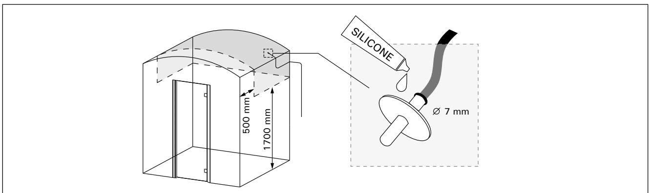
Figura 8. Cómo colocar el sensor de temperatura Figura 8. Posizionamento del sensore di temperatura
