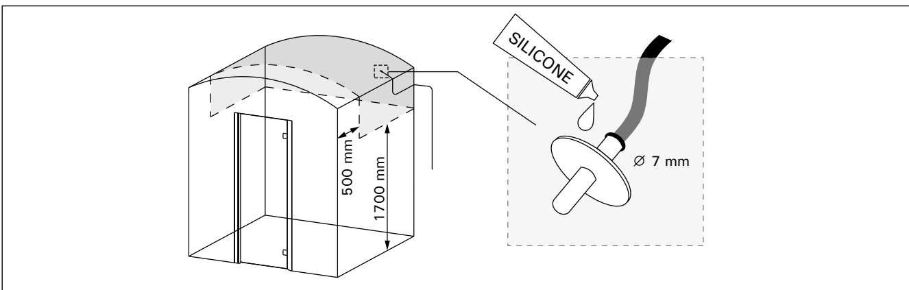
Figure 8. Placer le capteur de température Figuur 8. De temperatuursensor plaatsen
