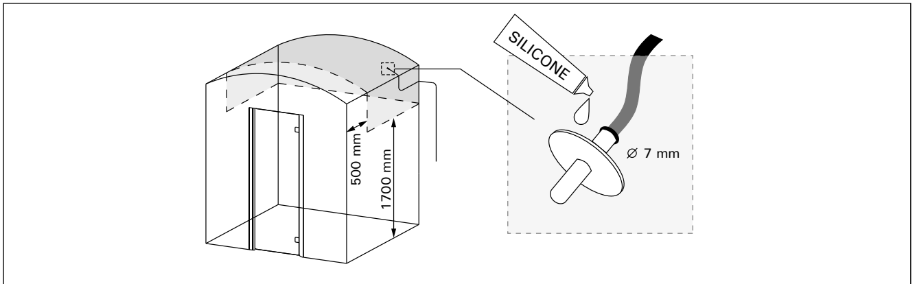
Kuva 8. Lämpöanturin sijoittaminen Bild 8. Placera temperatursensorn
