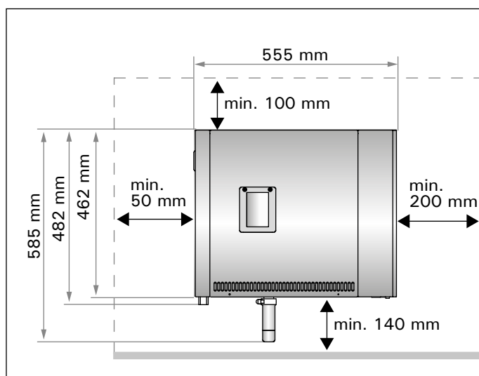
Figure 5. Mesures d'installation Figuur 5. Installatiemetingen
