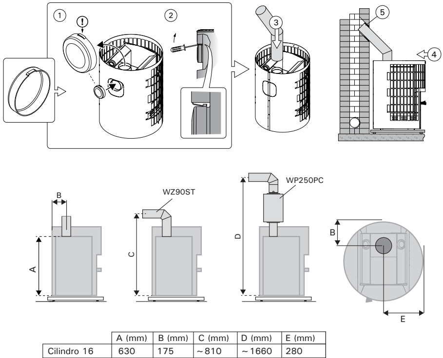
Figure 10. Raccordement du poêle à un conduit de fumée en maçonnerie par l'ouverture supérieure.
