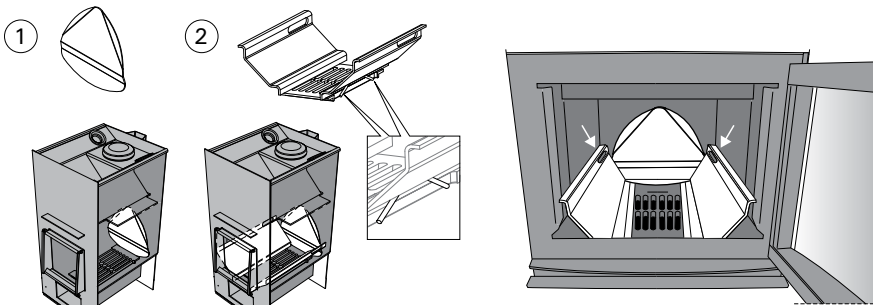
Abbildung 2. Verbrennungsluftleitbleche
