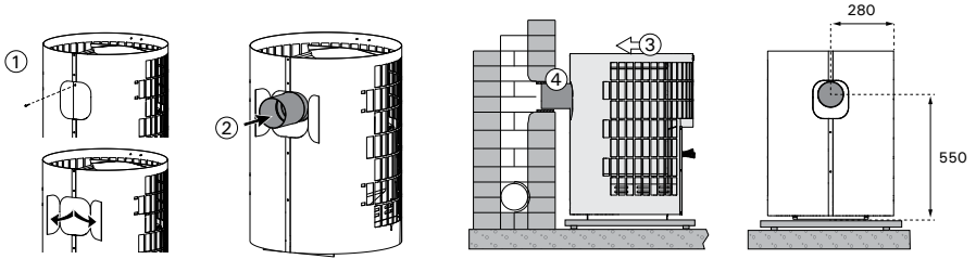
Abbildung 9. Anschluss des Saunaofens an einen gemauerten Rauchabzug durch die hintere Öffnung
