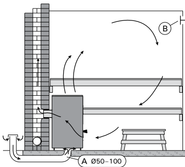
Abbildung 4. Schwerkraftlüftung
